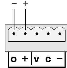
Sensorstromversorgung
