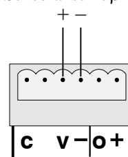
Sensoranschluß
