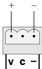
Sensoranschluß
